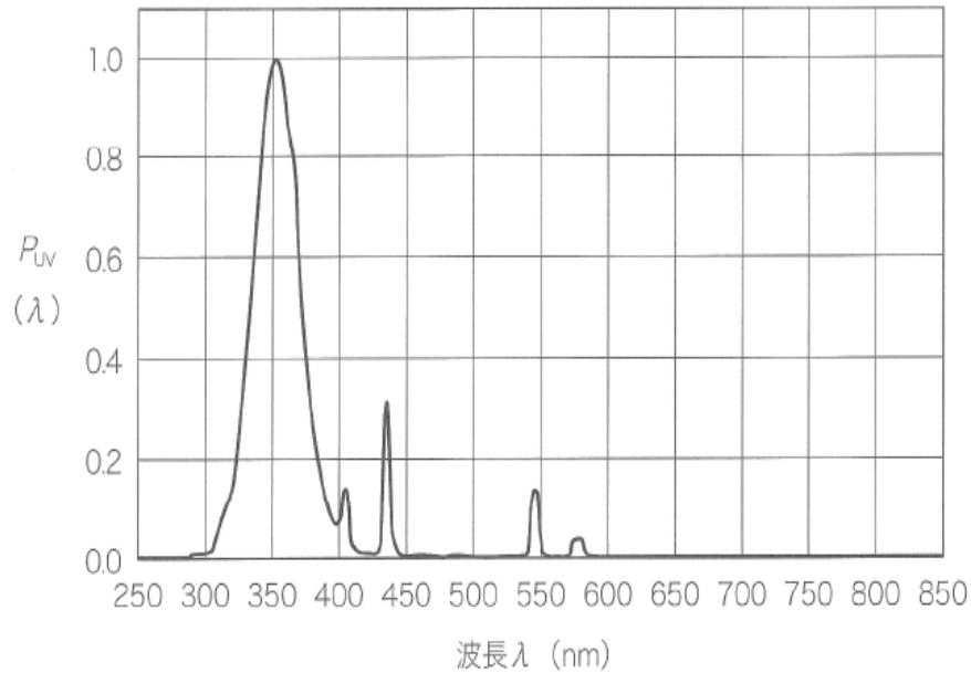
圖 1 為求紫外線響應特性 u 之輻射源的分光分布
