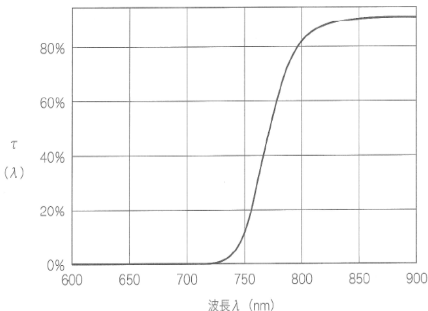
圖 3 為求紅外線響應特性 r 之 IR 濾光器之分光透過率 \tau(\lambda)
