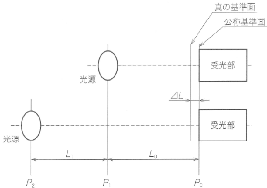
圖 D.1 受光基準面位置之測定說明圖
